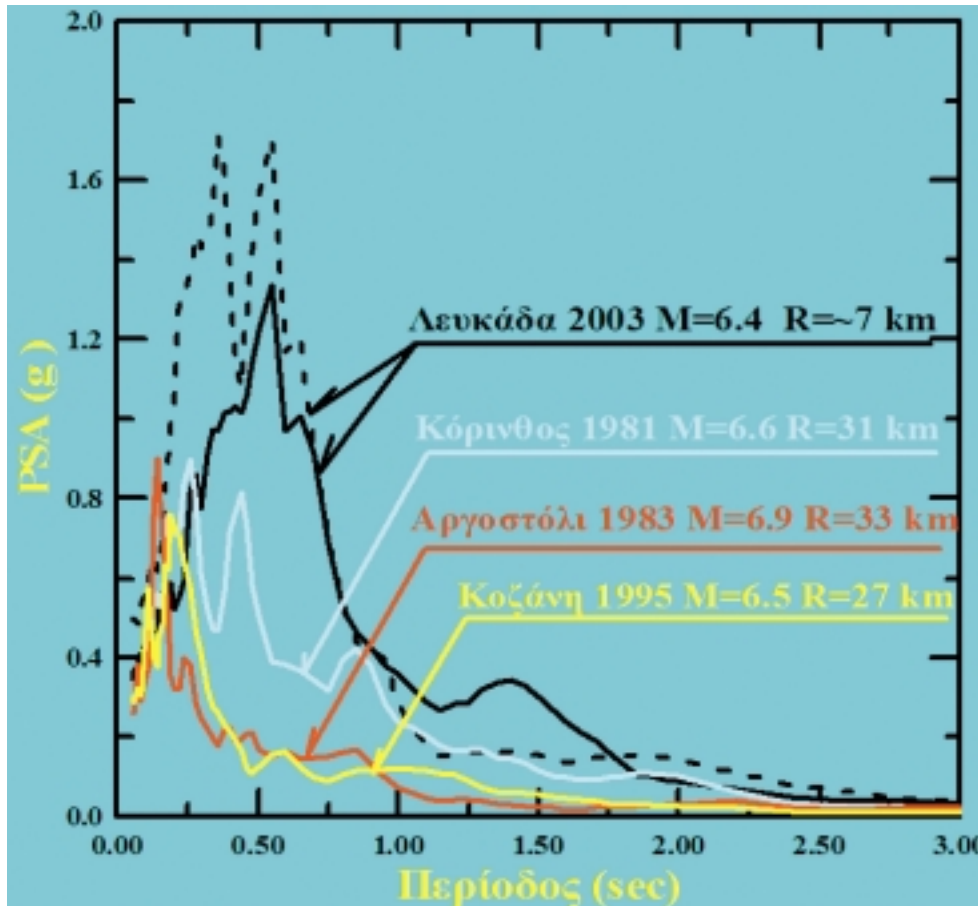
Σύγκριση Φασμάτων Απόκρισης PSA ( \xi=5\% ) Ισχυρών Σεισμών του Ελλ. Χώρου
